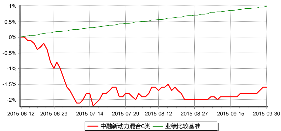
中融新动力混合C累计份额净值增长率与同期业绩比较基准收益率的 历史走势对比图 (2015年6月12日至2015年9月30日)
